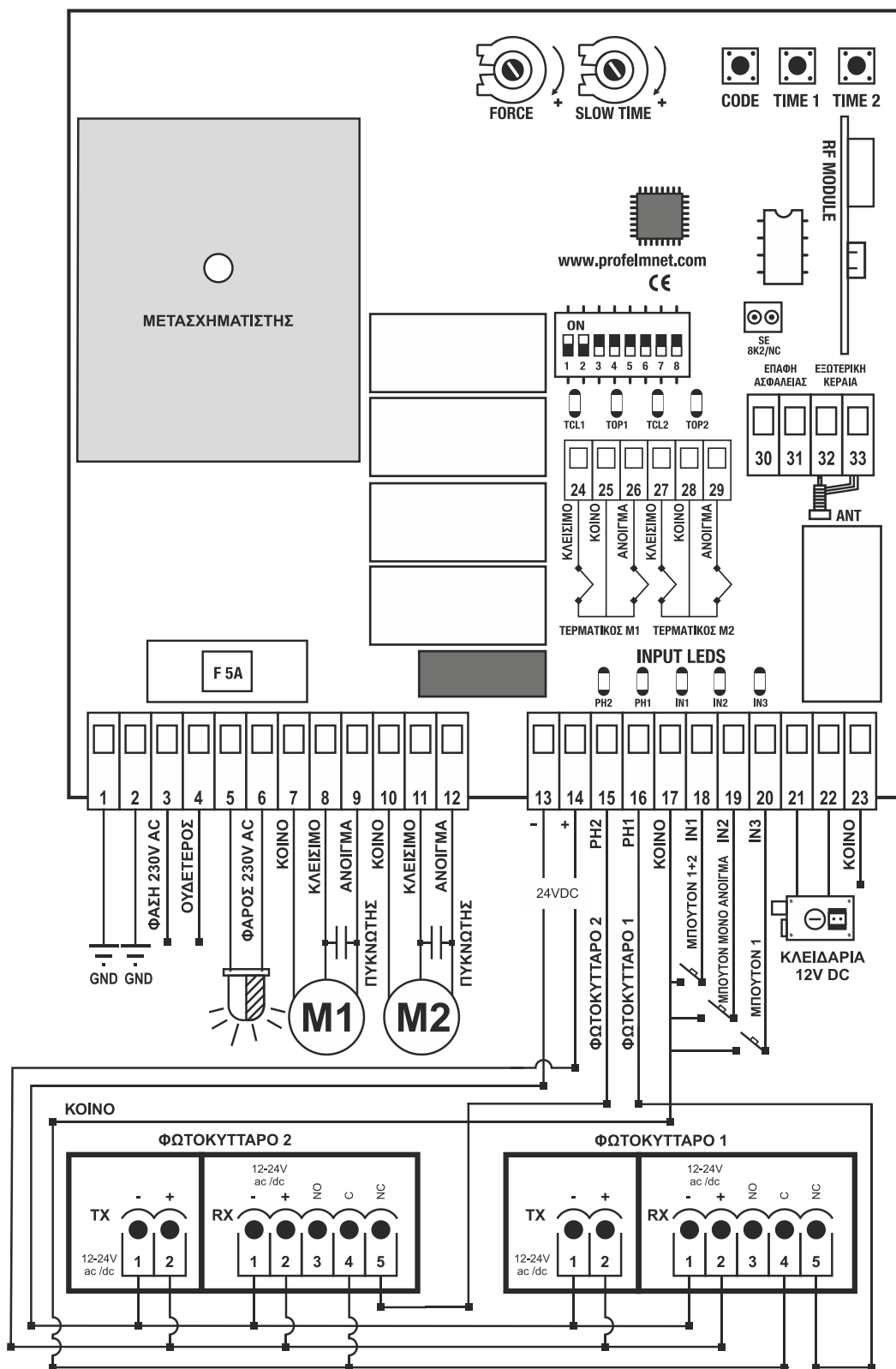
ΣΥΝΔΕΣΗ ΕΠΑΦΗΣ ΑΣΦΑΛΕΙΑΣ ΜΕ ΚΛΕΙΣΤΗ ΕΠΑΦΗ NC
